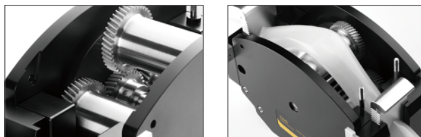
滚轮总成
